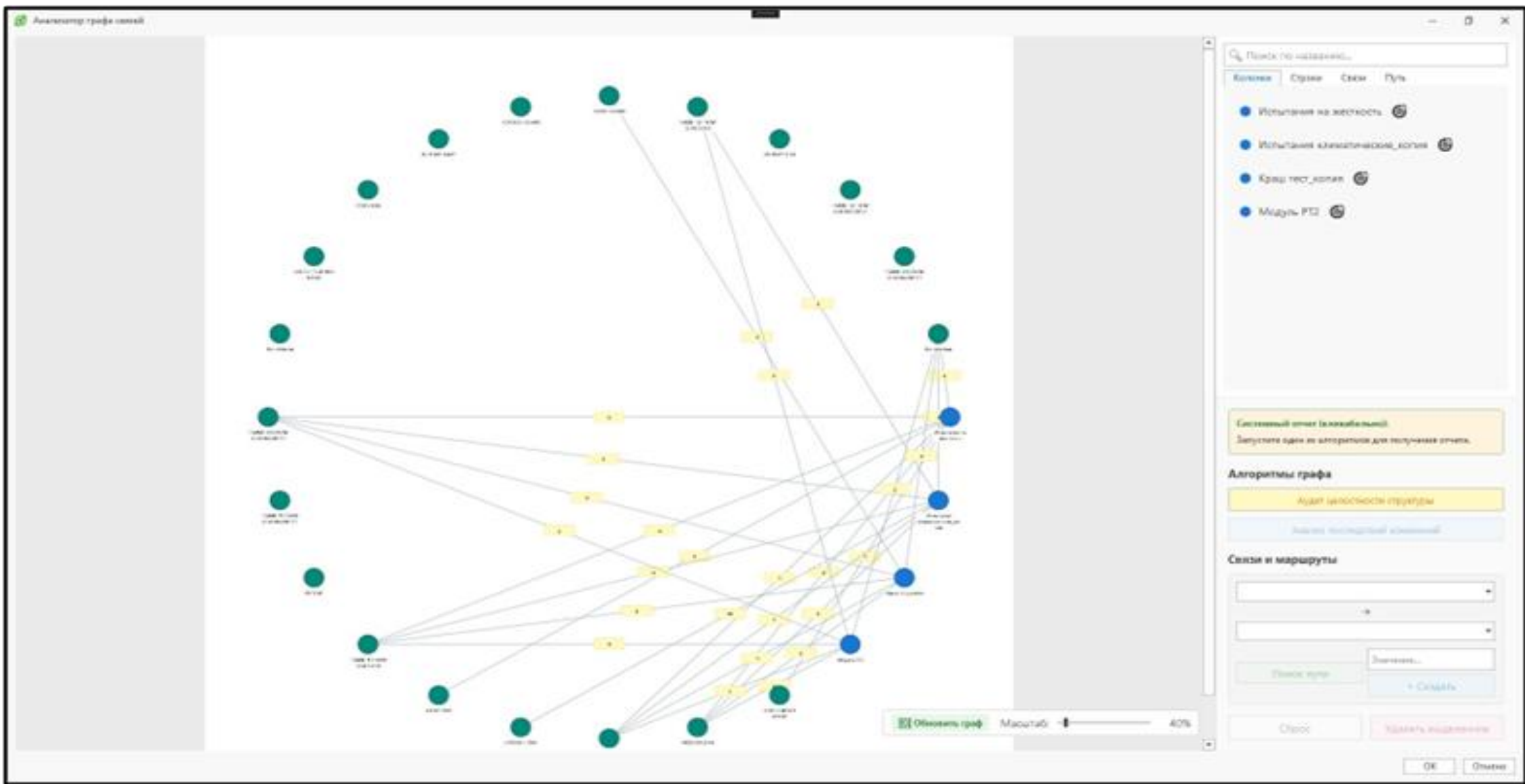
Визуализатор графа
